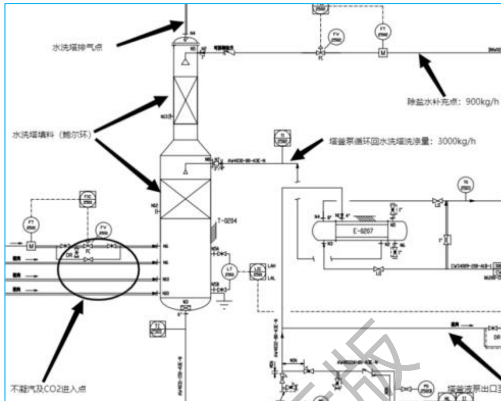
图 9.2.4-1 含氨废气水喷淋塔结构示意图
