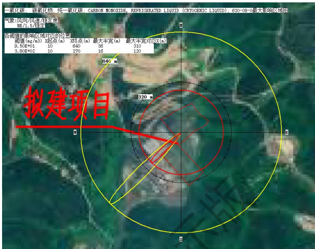
图 8.9.2-7 最不利气象条件下 CO 泄漏最大影响范围图
