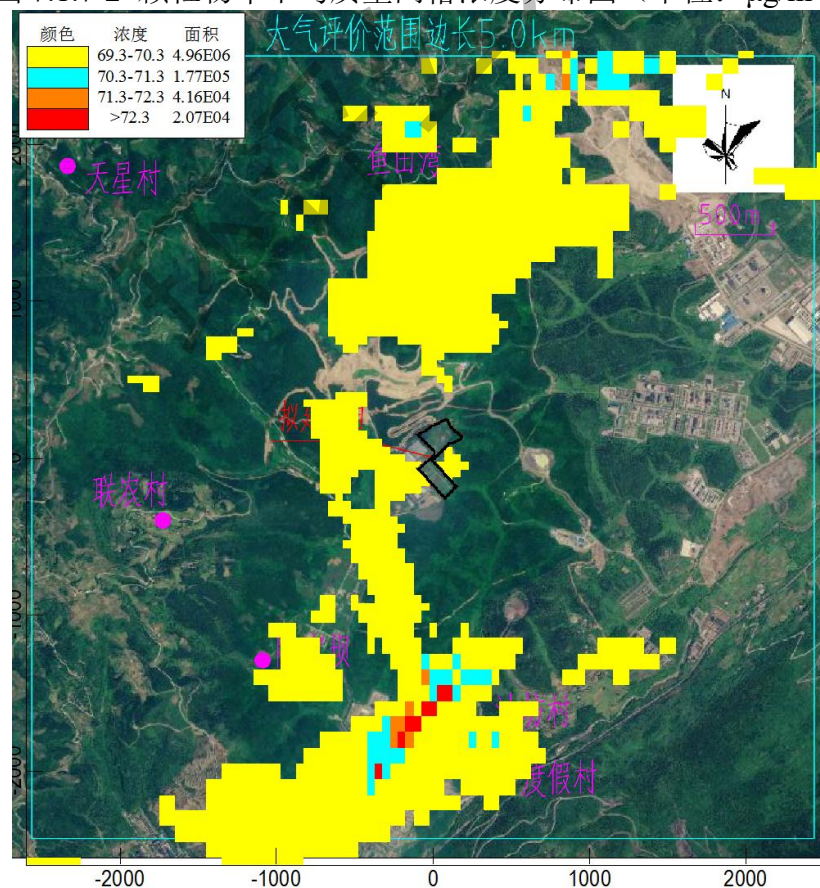
图 7.1.7-3 \text{PM}_{2.5} 95%保证率日平均质量网格浓度分布图 (单位: \mu\text{g}/\text{m}^3 )
