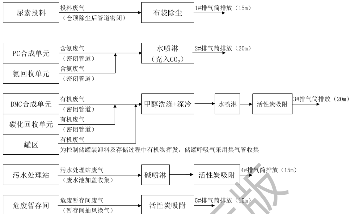
图 9.2.3-1 有组织废气收集、处理措施示意图
