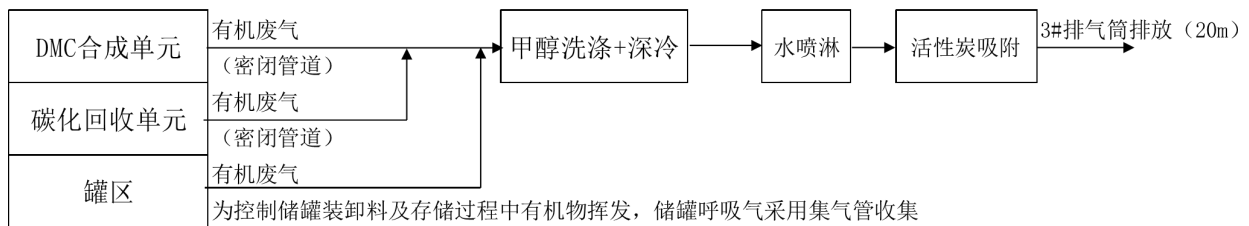
图 9.2.4-2 有机废气处理工艺流程示意图
