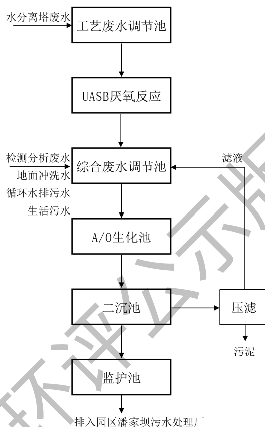
图 9.3.2-1 拟建项目污水处理工艺示意图
