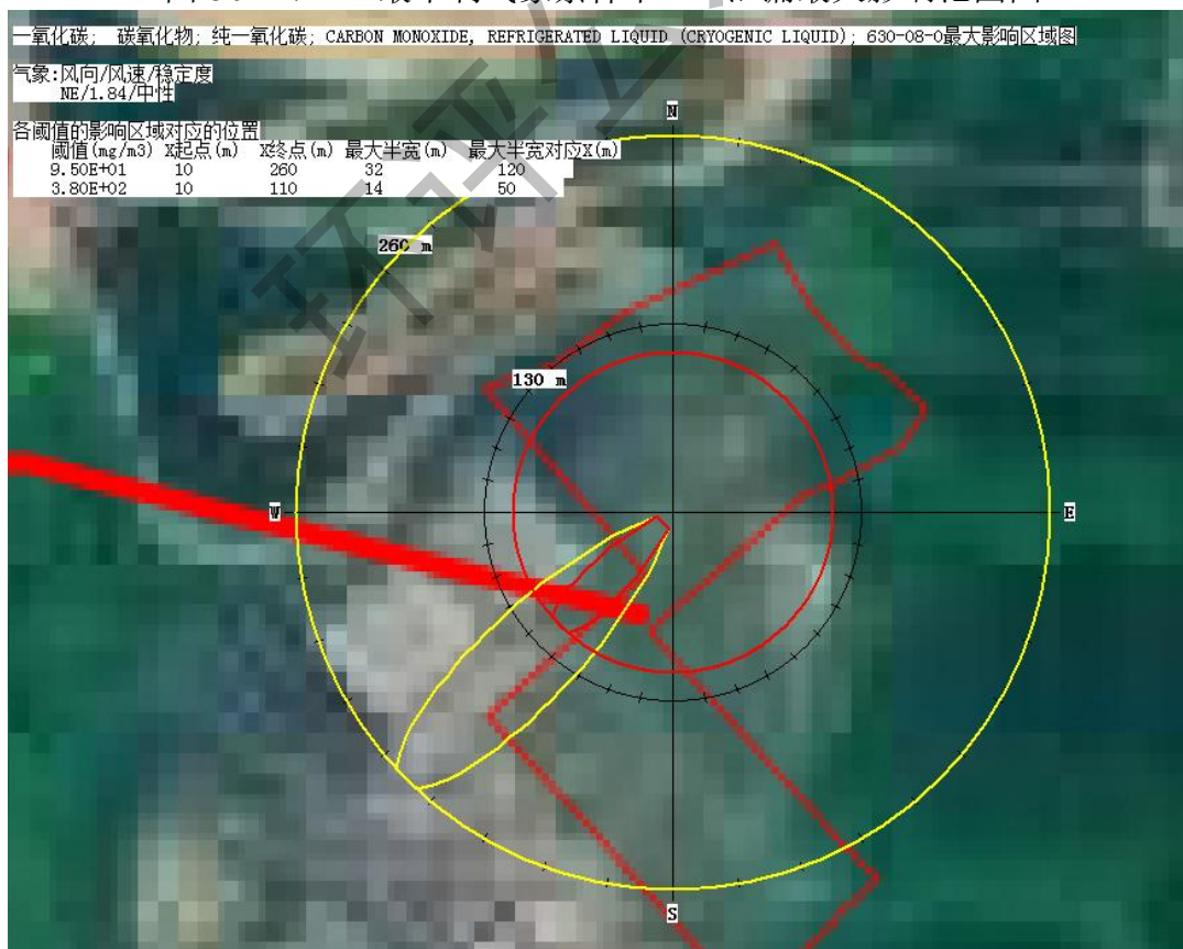
图 8.9.2-8 常见气象条件下风向不同距离 CO 浓度分布图
